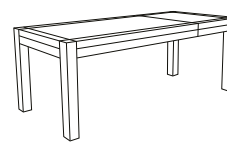
5ft Ext Leg Dining Table L202cm D90cm H77cm
